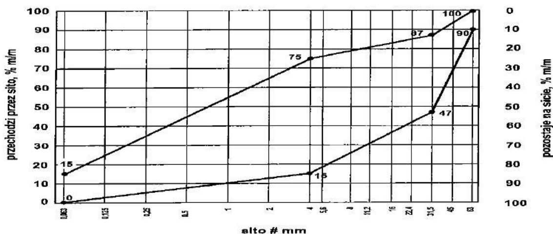
Rys. 6.7. Uziarnienie mieszanki niezwiązanej 0/63 do podłoża ulepszonego
